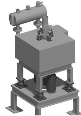
필터형 건식 철분 분리기 Filtered Dry Ferrous Powder Separator
