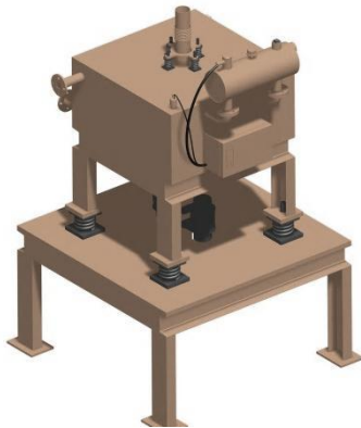
필터형 습식 철분 분리기 Filtered Wet Ferrous Powder Separator
