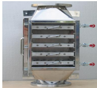
마그네트 바 유닛 Magnet Bar Unit
